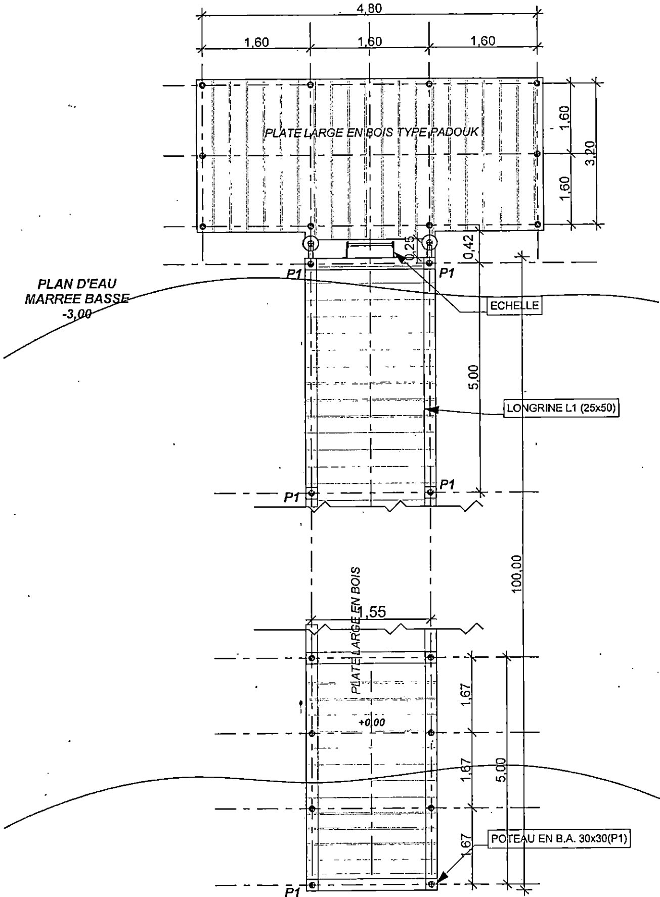
PLAN D'ENSEMBLE
